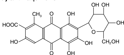
a) anthraquinone
