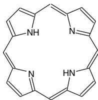
a) porphyrin
